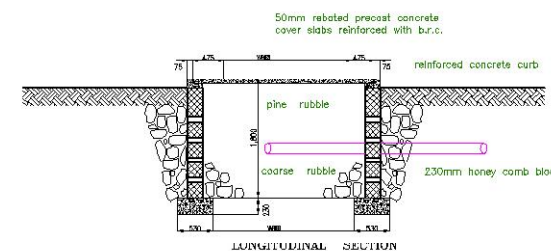
LONGITUDINAL SECTION
