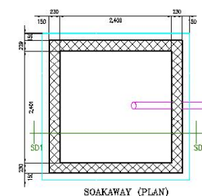
SOAKAWAY (PLAN)
